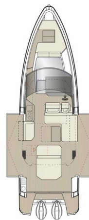
saxdor 400 gto layout
