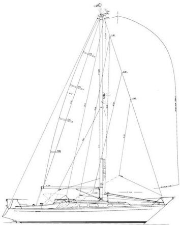
Segelplan
